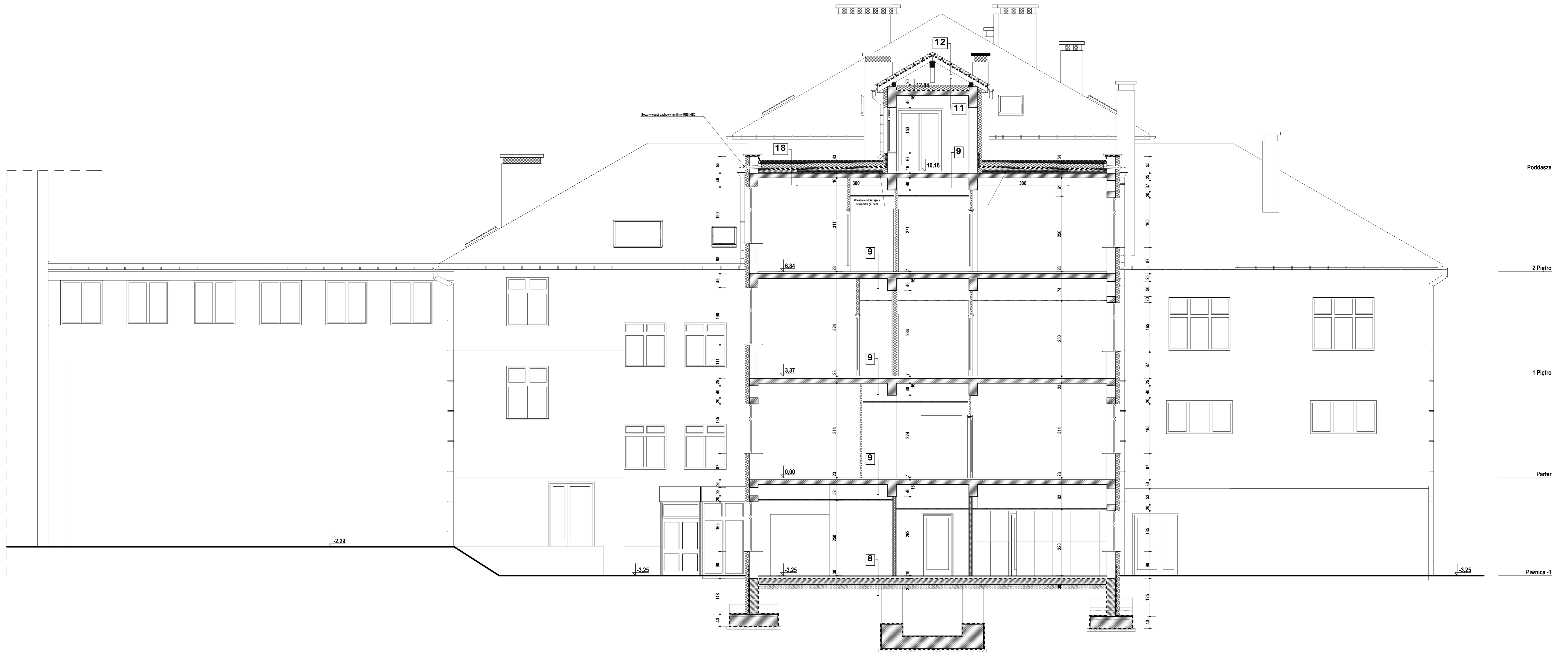
PRZEKRÓJ 5-5
